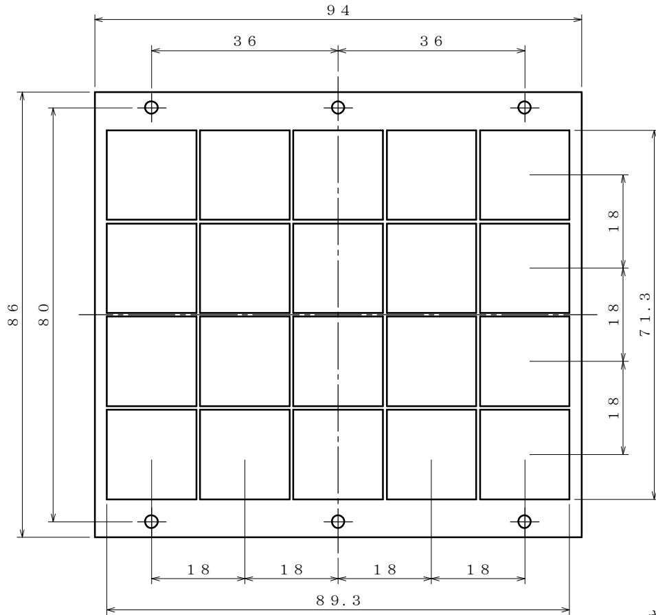
IKQT-45キーボード寸法図
