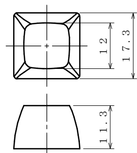
キートップ(QTT)寸法図
