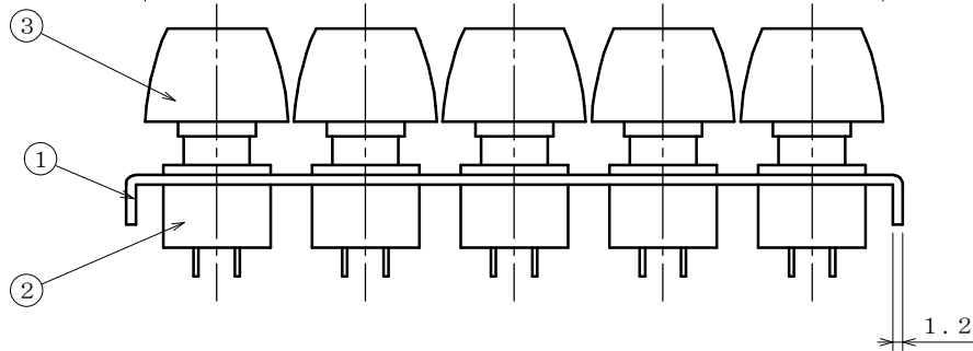
キートップ(QTT)寸法図
