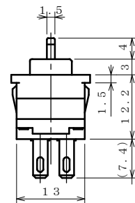
スイッチ (MM9-3) 寸法図・仕様
