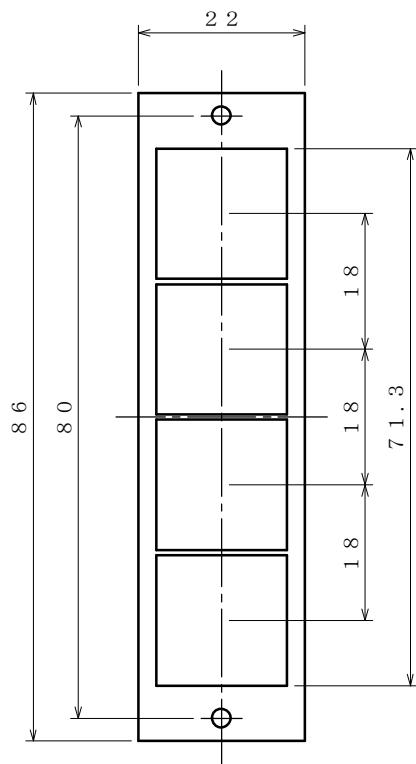
IKQ-41-3 キーボード寸法図
