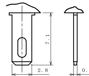
接触端子部詳細図
