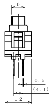
スイッチ (MM9-3) 寸法図・仕様
