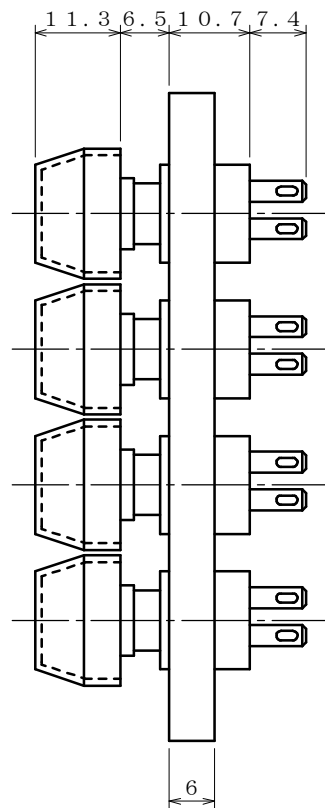
キートップ(QTC)寸法図
