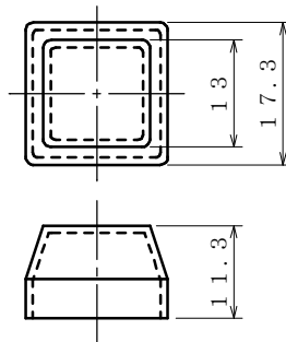
キートップ(QTC)寸法図
